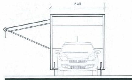
VISTA FRONTAL - TRAILER ESCALA: 1/75
