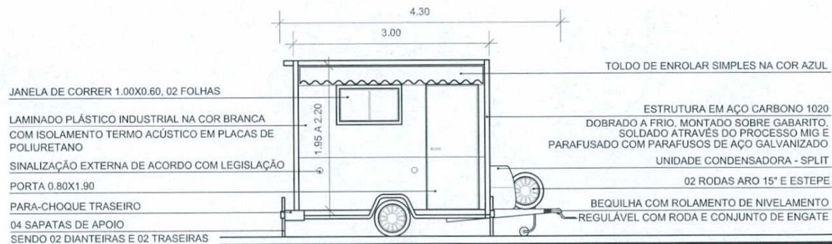
VISTA LATERAL DIREITA - ESPECIFICAÇÕES TRAILER ESCALA: 1/75
