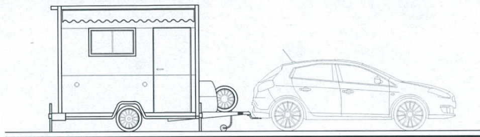
VISTA LATERAL DIREITA - TRAILER ESCALA: 1/75
