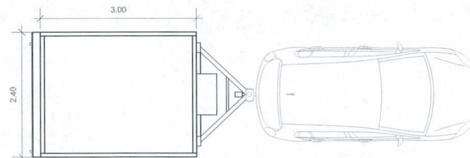
VISTA SUPERIOR - TRAILER ESCALA: 1/75
